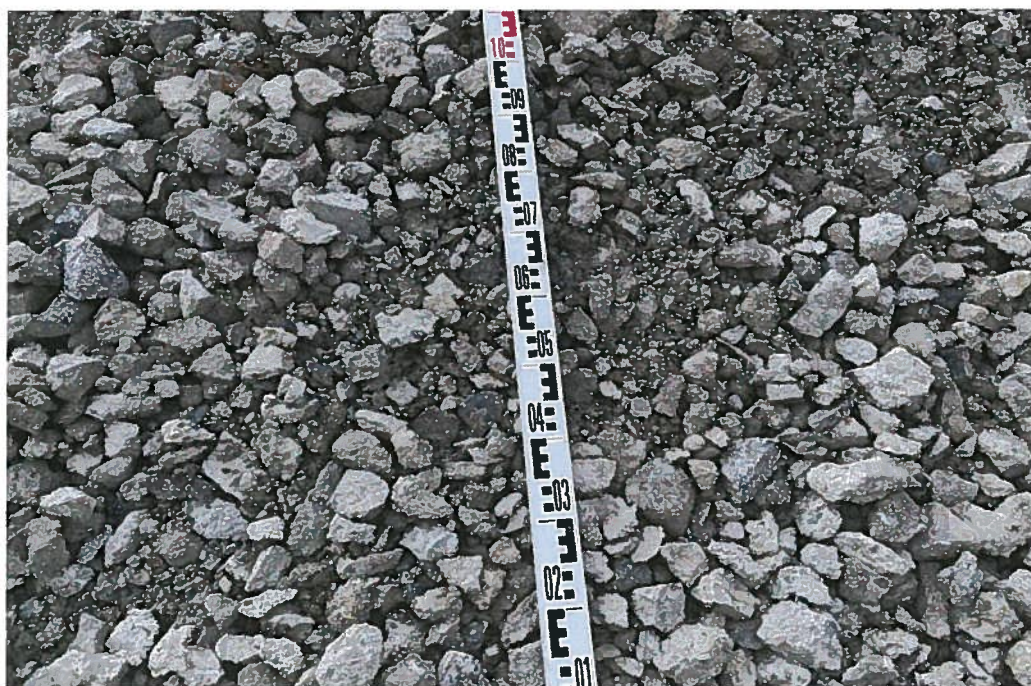
Foto 2: Detailaufnahme der recycelten Gesteinskörnung
